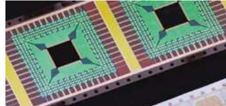
TAB/COF テープ連続電解 Ni/Au めっき
